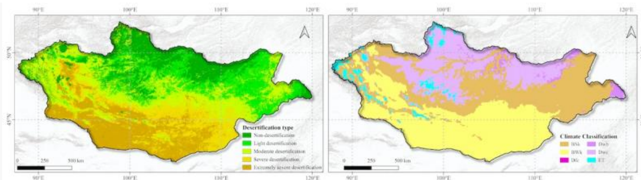
Карта, показывающая степень опустынивания и климатические зоны Монголии
