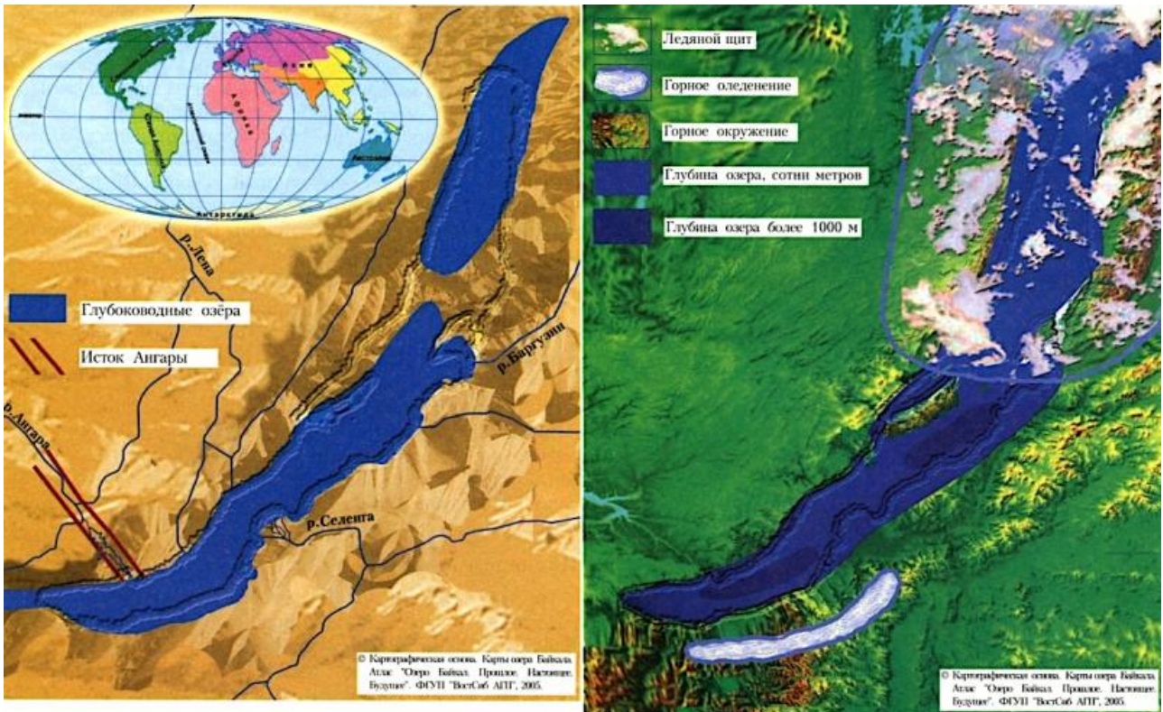
Схема расположения озёр на современном контуре Байкала 3–1 млн лет назад. Вверху слева – расположение материков на поверхности Земли 3 млн лет назад. Вверху справа – схема расположения озёр на современном контуре Байкала в период от 1 млн лет назад до настоящего времени.
