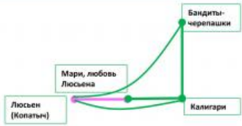
Вырожденный граф кино «Титаник» в «Смешарики: Начало»: 1) Разрушается связь Мари и Калигари 2) Умирает Мари – пропадает ее вершина со всеми связями 3) Повержены бандиты-черепашки – пропадают их вершина со всеми связями 4) ...
