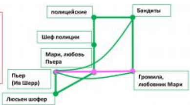
Вырожденный граф кино «Спаситель» в «Самородке»: 1) Разрушается связь Мари и Громилы 2) Умирает Пьер – пропадает его вершина со всеми связями 3) Умирают бандиты – пропадают их вершина со всеми связями 4) Умирает Громилла – пропадает его вершина со всеми связями
