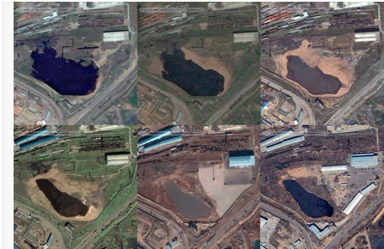
Эволюция фенольного озера с 2005 по 2023 год
