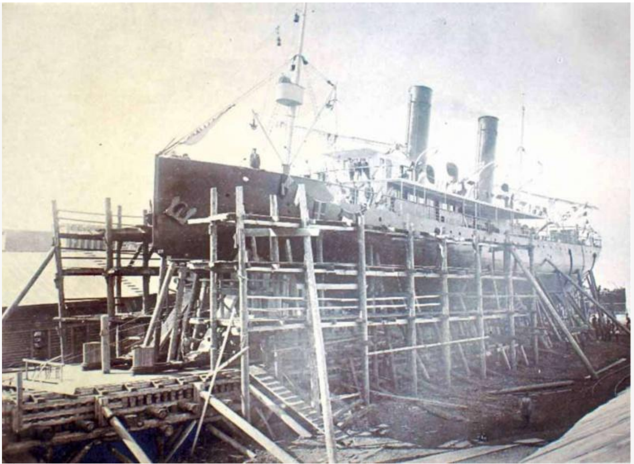
Сборка ледокола «Ангара»
